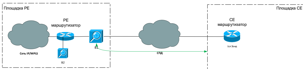
Рис.2 Типовые схемы подключения зондов на площадке типа PE
